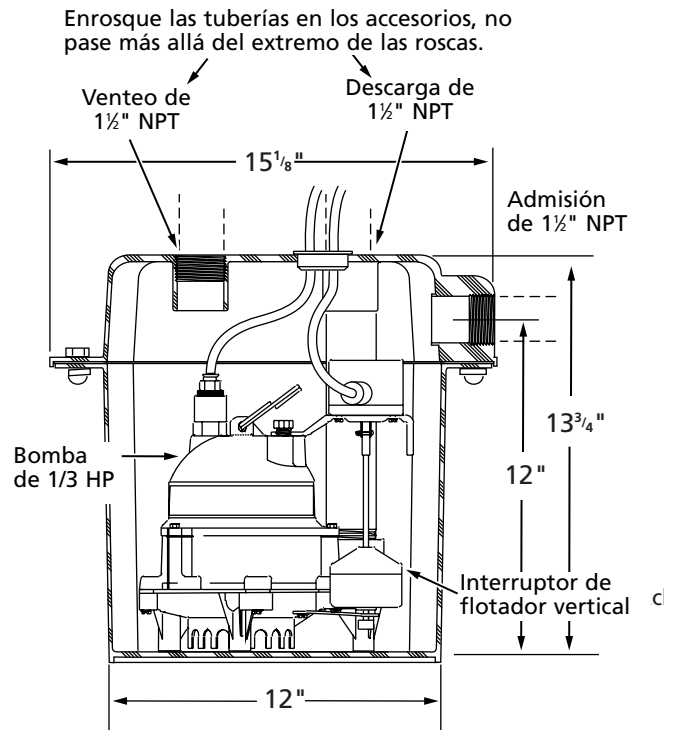
Figura 7 – Dimensiones del Sistema de Desagüe con Plomería
